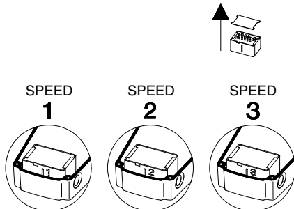
Fig. 8 Speed switch module
