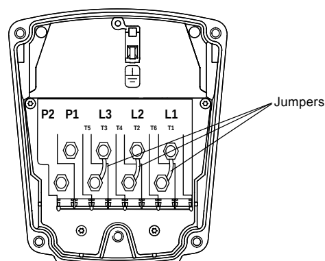
Fig. 11 3 x 460 V & 575 V terminal box
