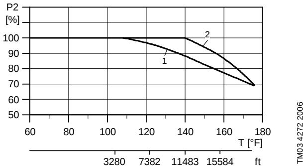
Fig. 1 Relation entre débit moteur ( P_2 ) et température ambiante/altitude
