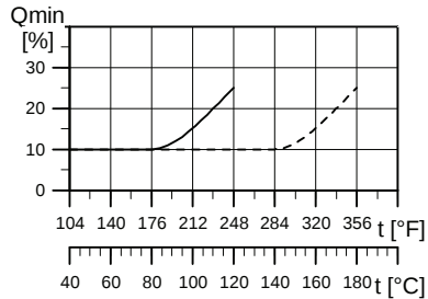
Fig. 5 Débit minimum
