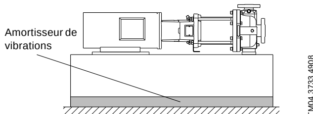
Fig. 10 Pompe sur amortisseur de vibrations
