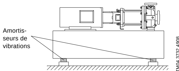
Fig. 9 Pompe sur amortisseur de vibrations
