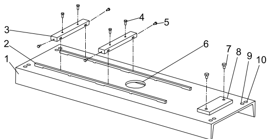
Fig. 11 Plataforma de base Grundfos
