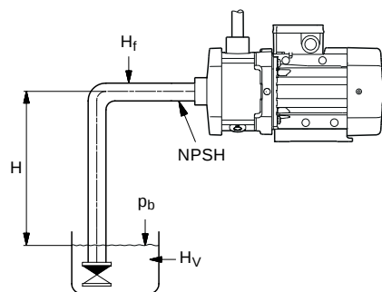
Fig. 13 Presión mínima de entrada (NPSH)
