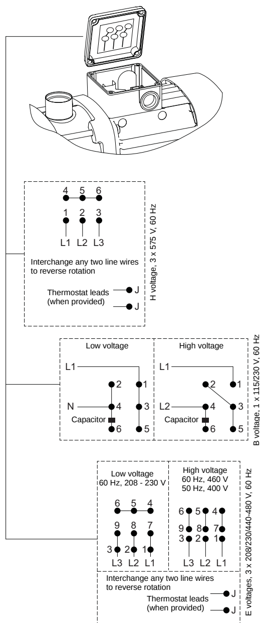
Fig. 10 Wiring diagram
