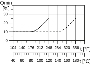
Fig. 5 Débit minimum
