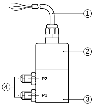
Fig. 68 DPI sensor
