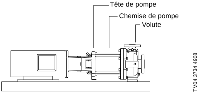
Fig. 12 Surfaces potentiellement chaudes sur une pompe CR-H et CRN-H
