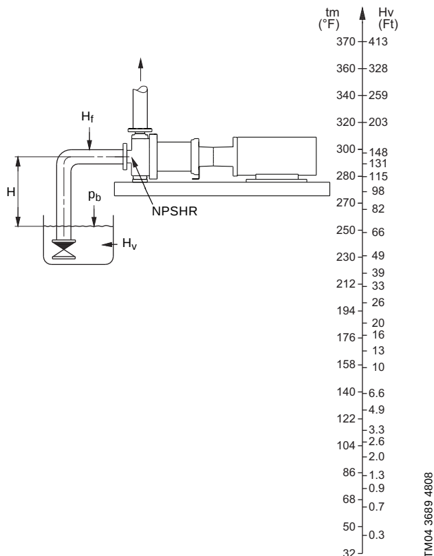
Fig. 4 Presión mínima de entrada – NPSHR
