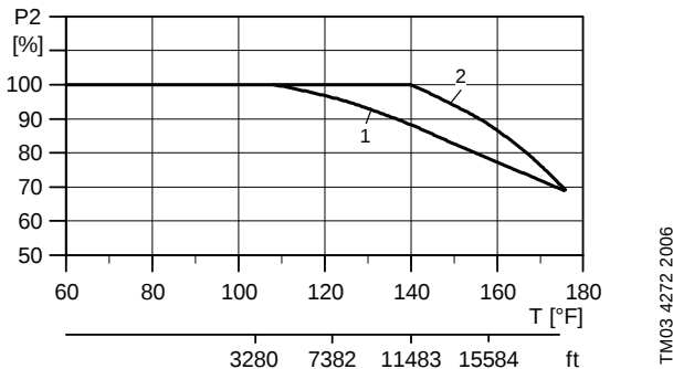
Fig. 1 Relación entre la potencia del motor ( P_2 ) y la temperatura ambiente / altitud
