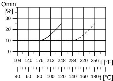
Fig. 5 Débit minimum
