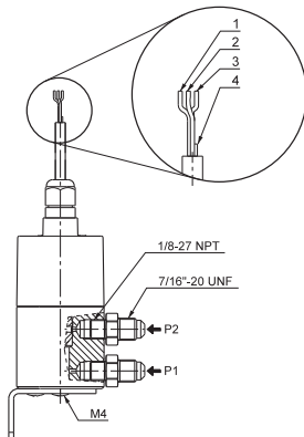
Fig. 70 Wiring
