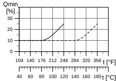
Fig. 5 Débit minimum
