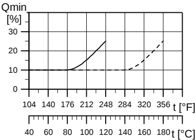
Fig. 5 Débit minimum
