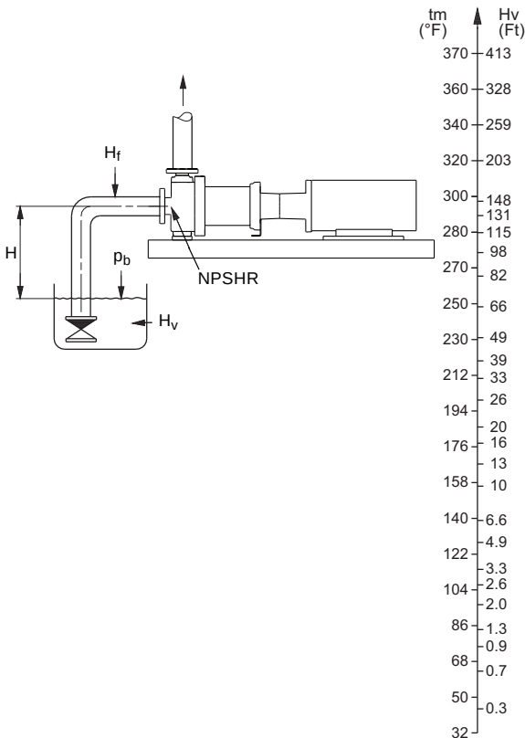
Fig. 4 Pression d'entrée minimale – NPSHR
