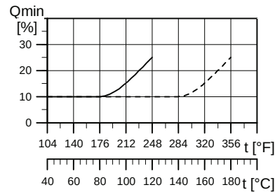
Fig. 5 Débit minimum
