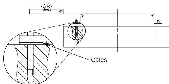
Fig. 8 Alignement avec cales
