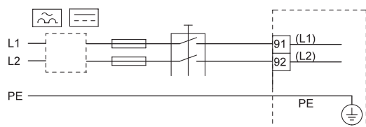
SmartFlo wiring diagram
