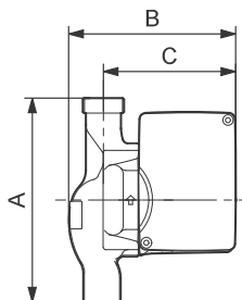
UP 15-10 BUC7, UP 15-10 BUC7/LC, UP 15-10 BUC7/TLC
