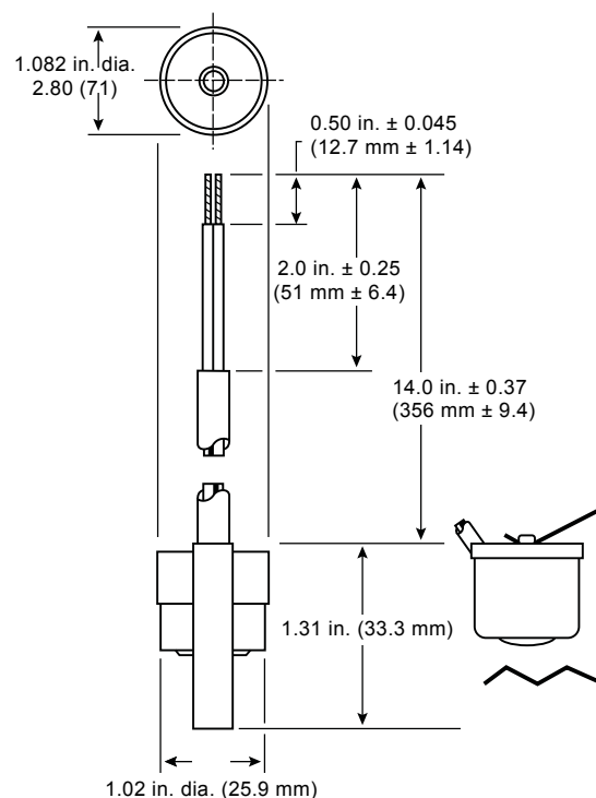
Fig. 10 Aquastat dimensions
