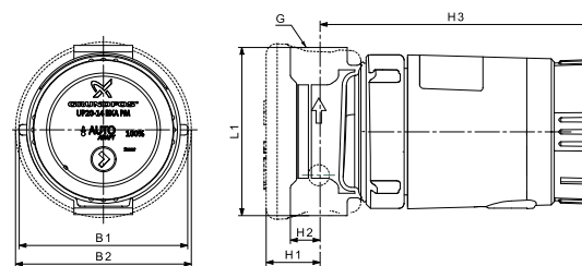
UP 10-16 A PM BU
