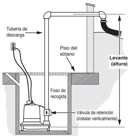
Figura 7 – LEVANTE (ALTURA): El levante (la altura) es la distancia vertical efectiva a la cual la bomba levanta el agua. Cuanto más alto sea el levante, más bajo será el flujo.
