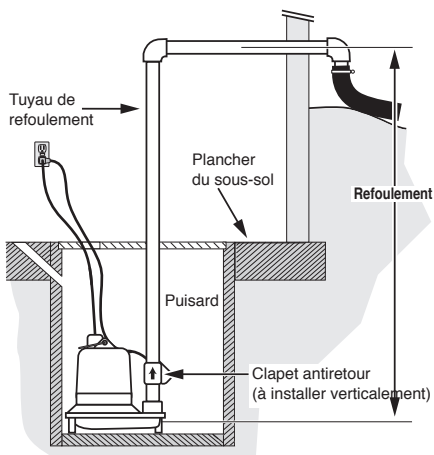
Figure 7 – REFOULEMENT : C’est la distance verticale à laquelle la pompe refoulera l’eau. Plus le refolement est haut, moins la pompe débite.
